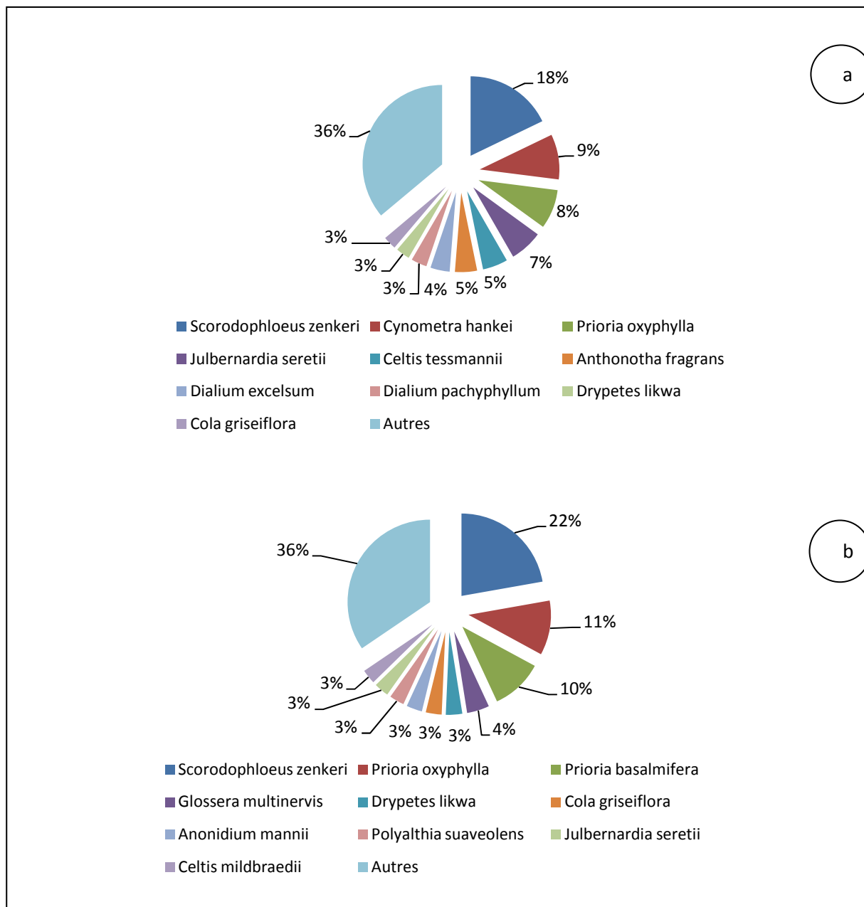
Figure 4.4 : Dominance relative des espèces inventoriées au sein deux peuplements (a : premier peuplement et b : deuxième peuplement)
