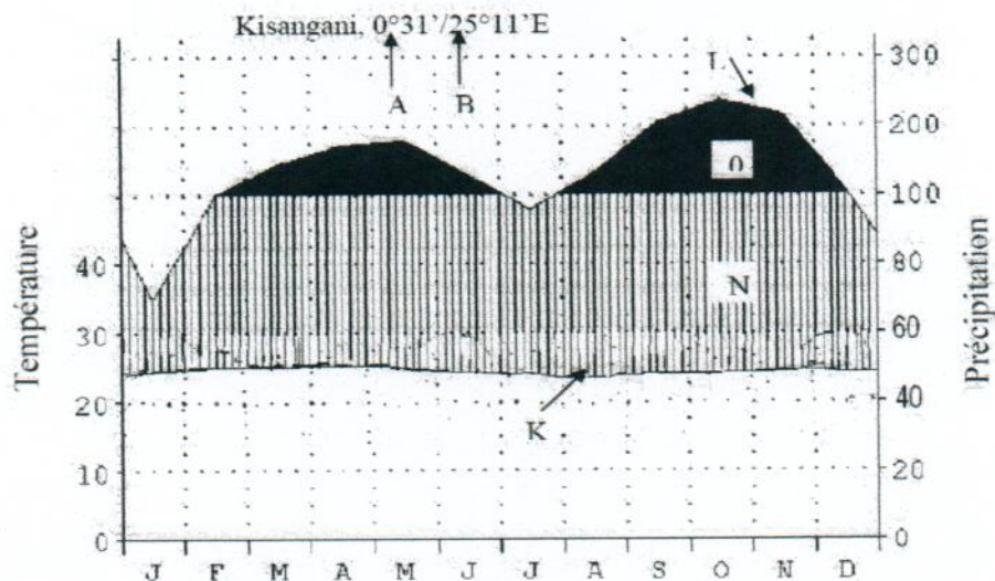
Figure 2.2 : Diagramme Ombrothermique de Kisangani (source : Nshimba, 2008)
