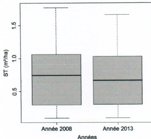
Figure 3.3 : Dispersion des valeurs des surfaces terrières de l'espèce Scorodophloeus zenkeri pour les années 2008 et 2013. La boîte représente l'intervalle dans lequel sont regroupés 50 % des surfaces terrières et la barre épaisse à l'intérieur de la boîte indique la surface terrière moyenne ; la barre basse indique la surface terrière minimale, la barre haute indique la surface terrière maximale
