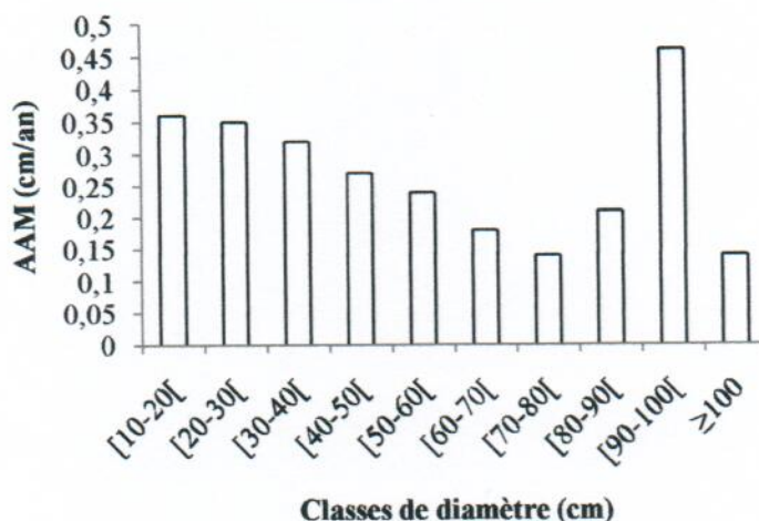
Figure 3.1 : Accroissements annuels moyens en fonction des classes de diamètre
