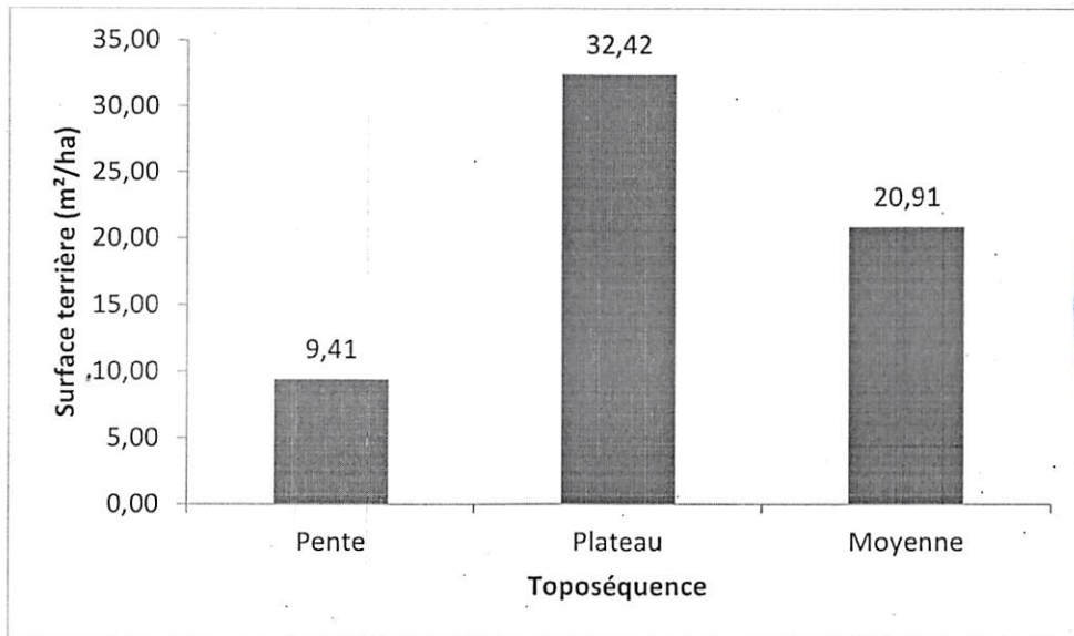
Figure 17 Surface terrière dans les toposéquences étudiées
