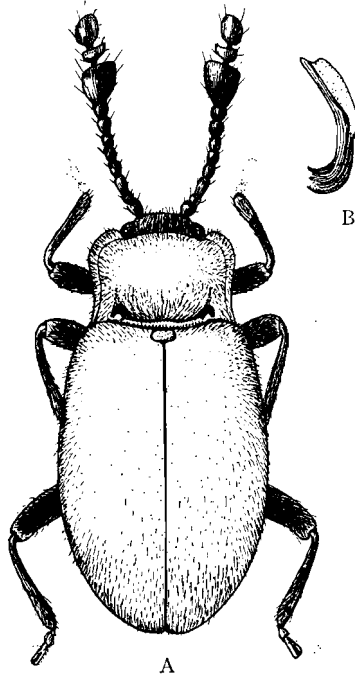
FIG. 8. — A. Danaë gracilis sp. n. B. Aedeagus.
