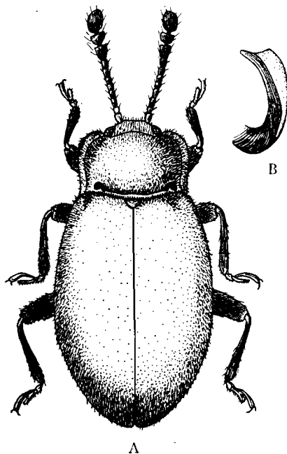
FIG. 11. — A. Danaë parvicornis sp. n. B. Ædeagus.
