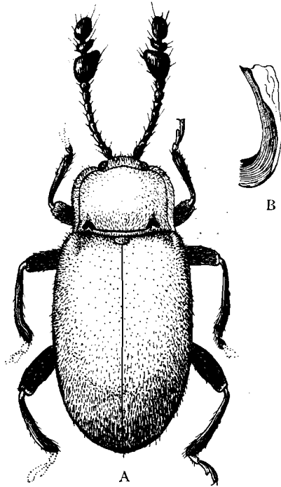
FIG. 6. — A. Danaë valga sp. n. B. Aedeagus.
