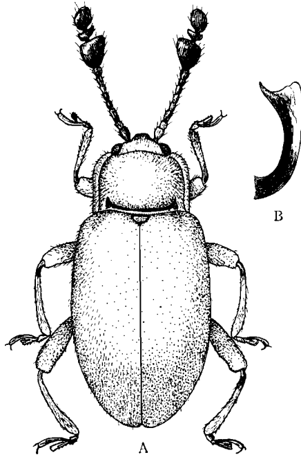
FIG. 5. — A. Danaë macra sp. n. B. Edeagus.
