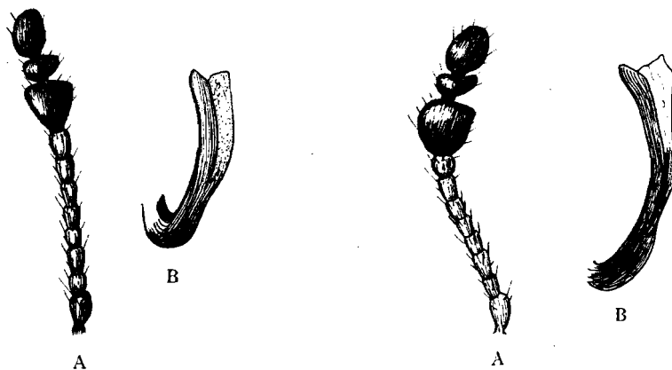
FIG. 12. — Danaë damnifica sp. n. A. Antenna. B. Aedeagus.
