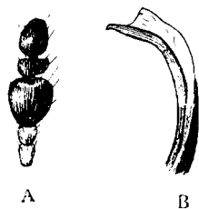
FIG. 14. — Danaë semicornis sp. n.
