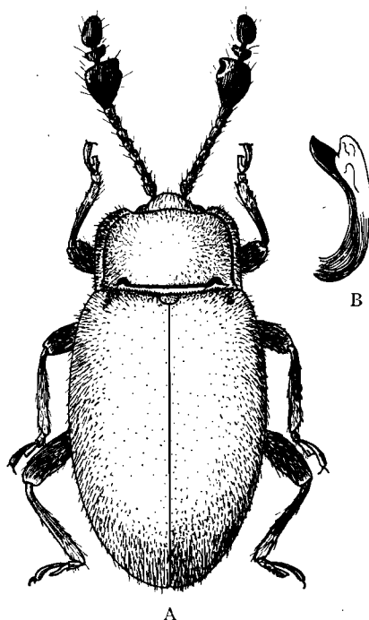
FIG. 7. — A. Danaë laticollis sp. n. B. Edeagus.
