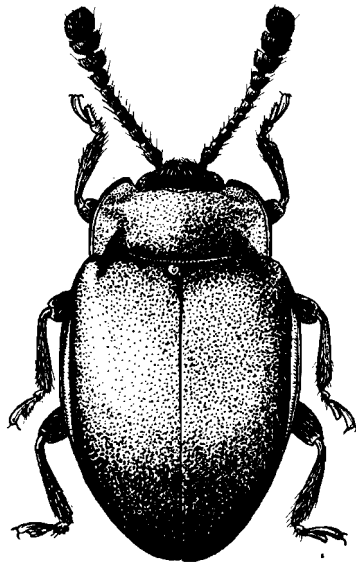
FIG. 1. — Mycetina rubescens sp. n.
