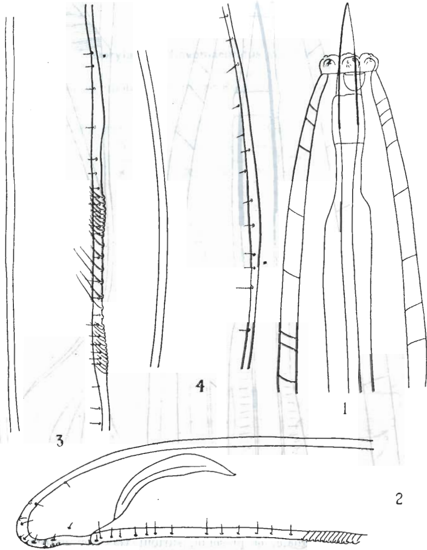
FIG. 3a. — Dorylaimus parhomalopapillatus n. sp.
