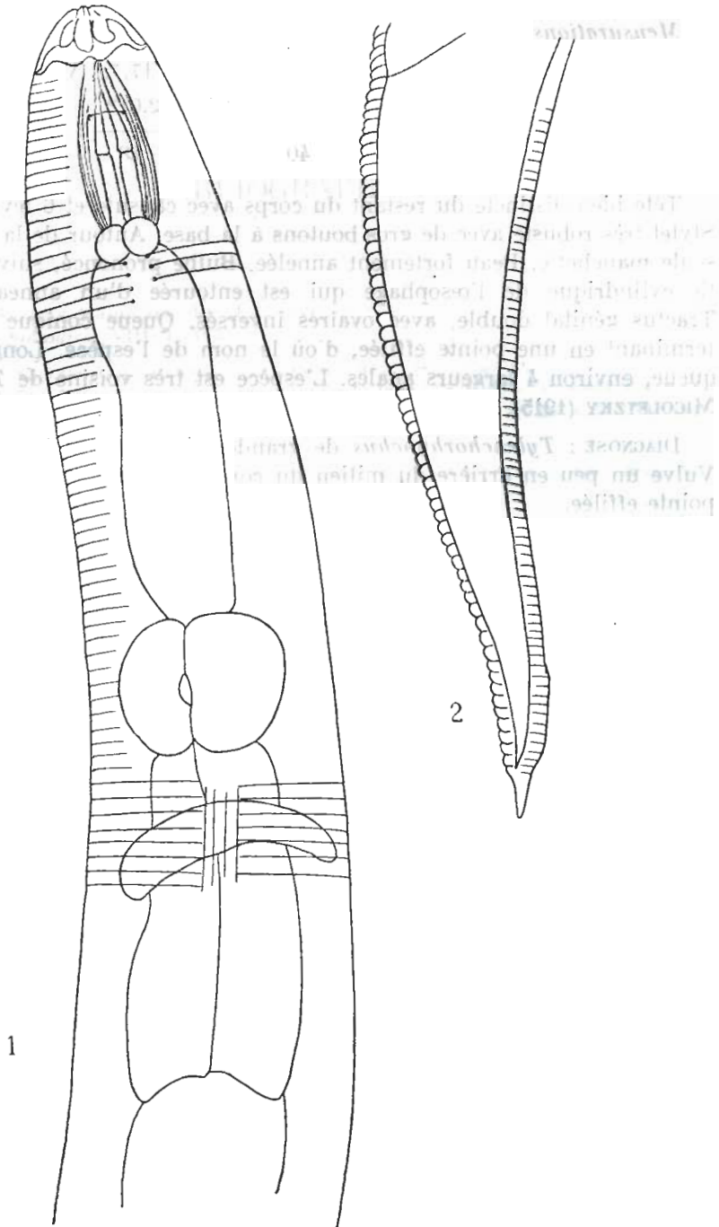
FIG. 7. — Tylenchorhynchus spinicaudatus n. sp.
