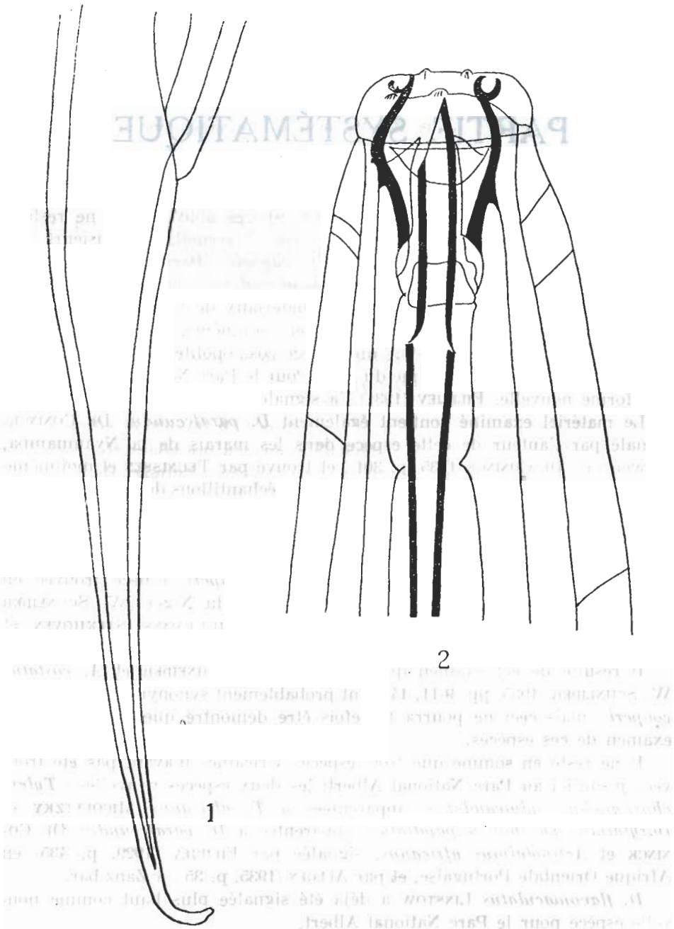
FIG. 1. — Actinolaimus africanus FILIPJEV.
