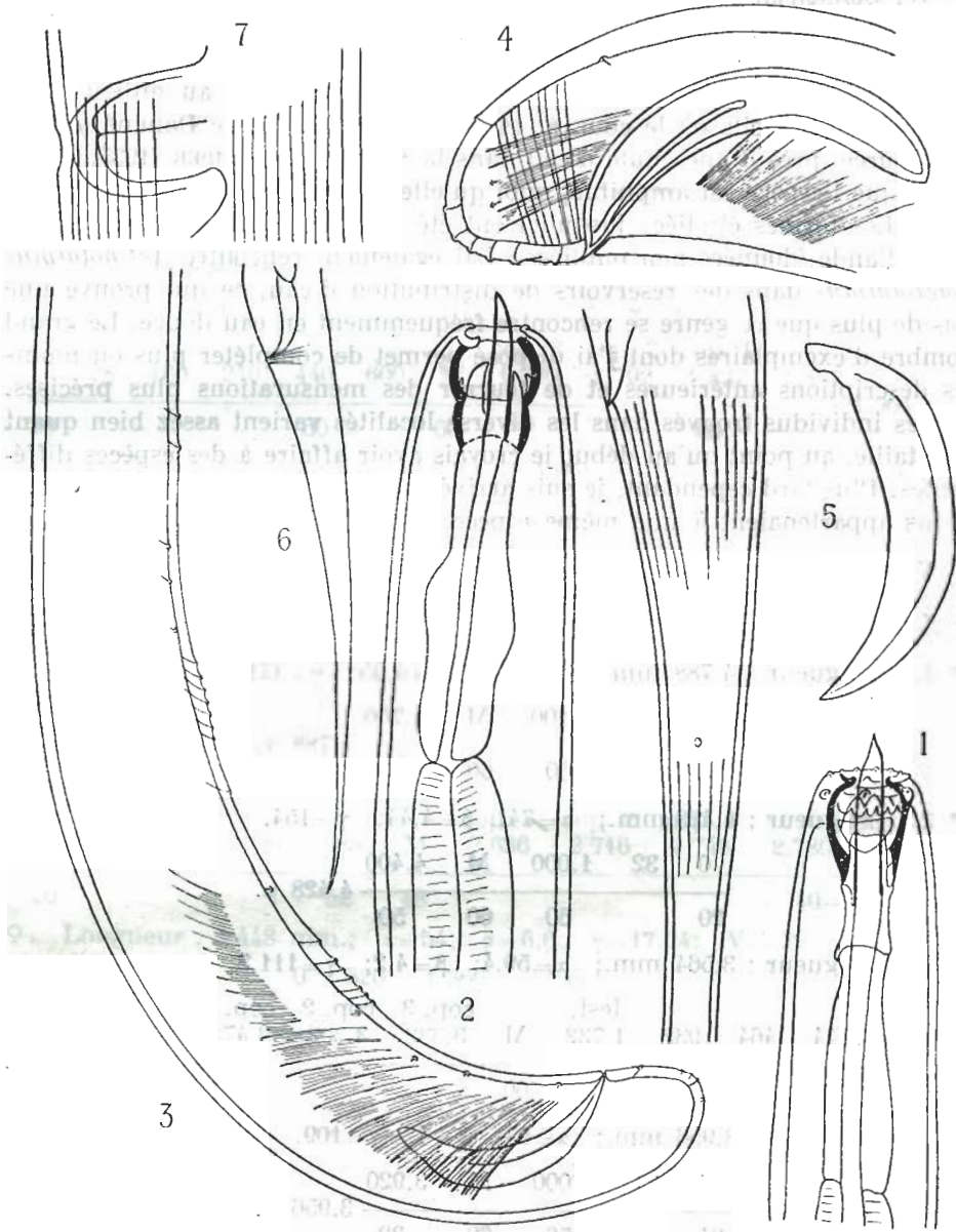
FIG. 2a. — Actinotaimus omer-cooperi FILIPJEV.
